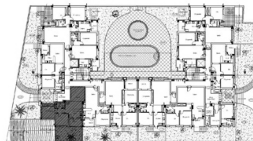
PLAN RDC
